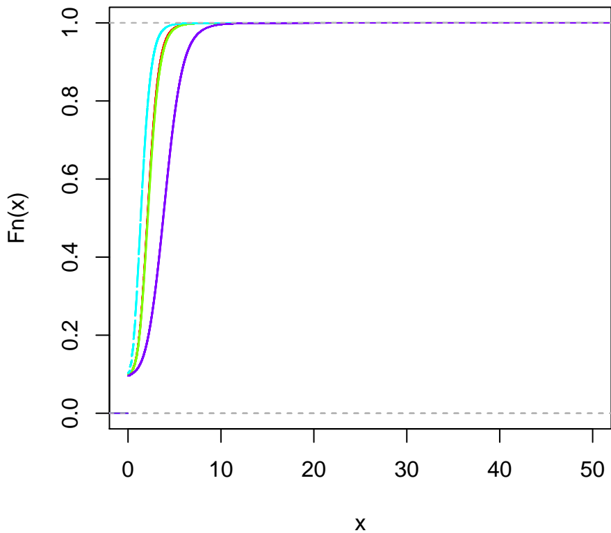
ecdf(df_data$gfp_input)
